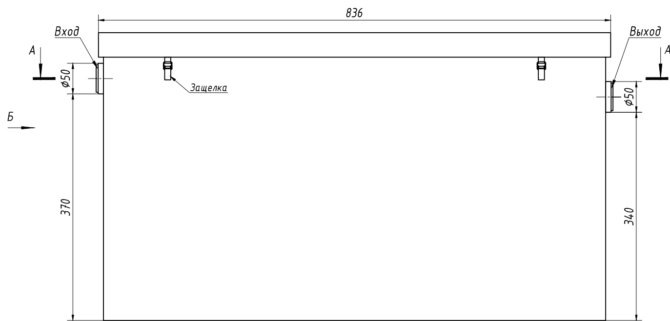
Вид спереди
