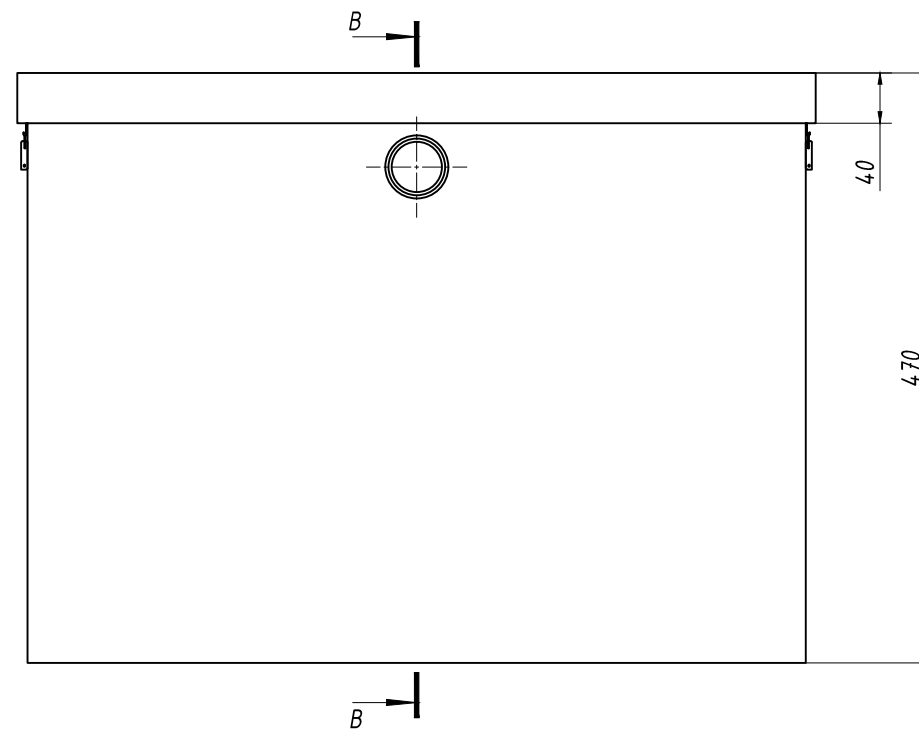
Вид Б
